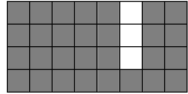
“EXOR”
